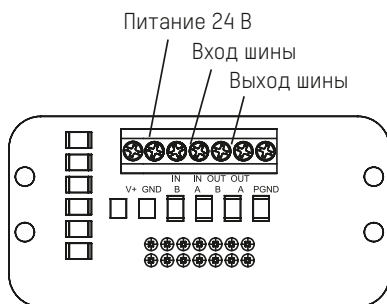
Клеммная колодка энкодера
