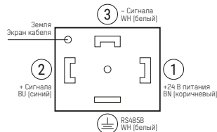
Разъем NM04
