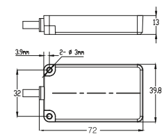
KTSR-A-H-MR-P4013
