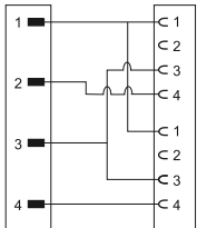
M12 A-CODE
