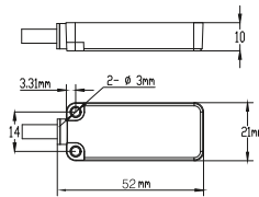
KTSR-A-H-MR-P4013
