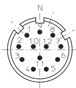
12-пиновый разъем
