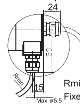
Cable output
