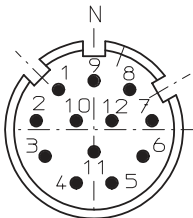
TMSP1612F
