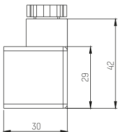
HM04: Прямоугольный разъем по DIN3650-A/ISO4400, 4-пин (штекер)
