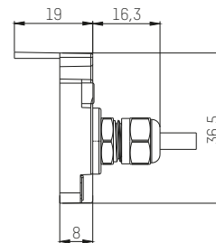
PRxx, PAxx: Герметичный ввод
