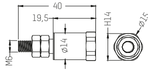
Укороченное универсальное соединение (опция)
