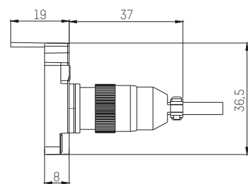
SM05: Авиационный разъем GB11918-2014 IP67, M18, 5-пин (гнездо)
