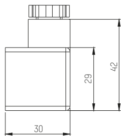
HM04: Прямоугольный разъем по DIN3650-A/ISO4400, 4-пин (штекер)
